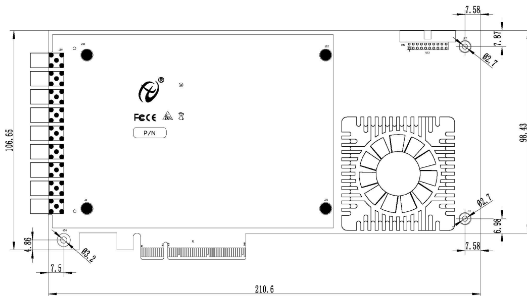
图 3-2-1 PCIe858xM 板卡尺寸图
