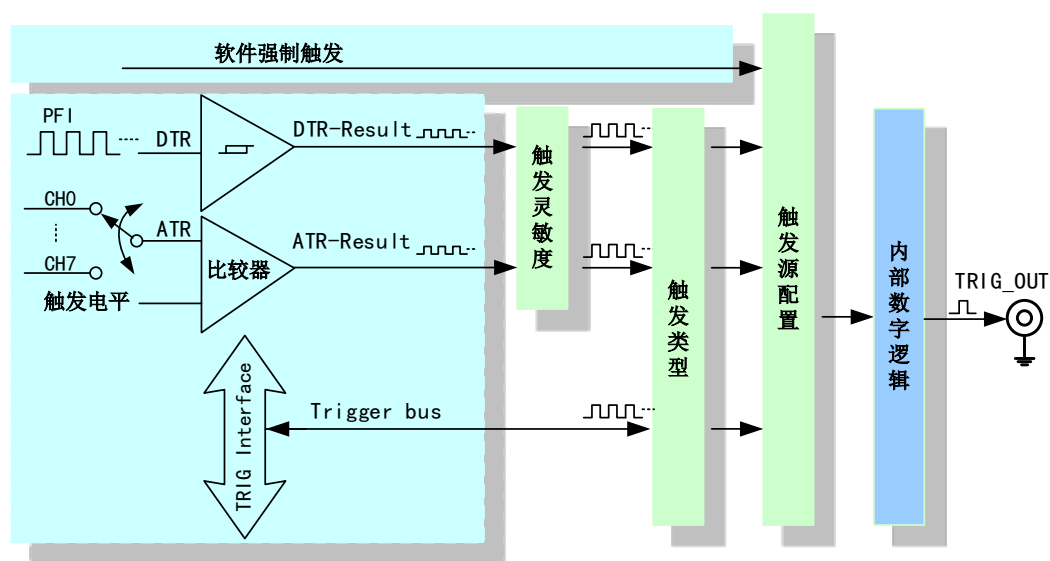
图 4-8-1 AI 触发功能框图
