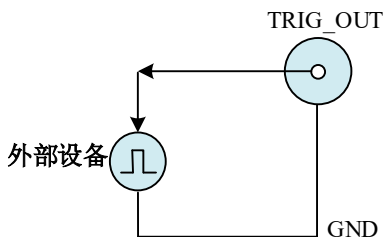
图 4-8-10 触发信号输出连接
