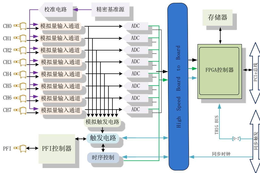
图 3-1-1 PCIe858xM 系统框图
