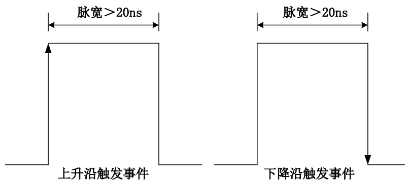
图 4-8-8 脉宽最小值图
