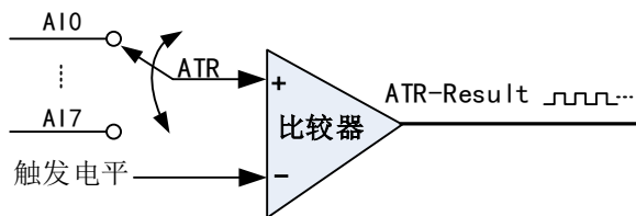
图 4-8-5 比较器
