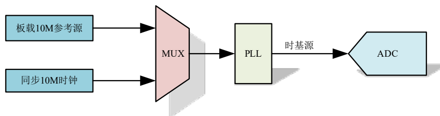
图 4-7-1 时基源框图
