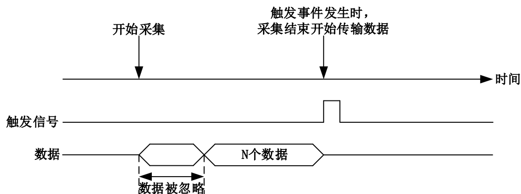
图 4-9-2-4 预触发
