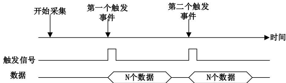
图 4-9-2-7 后触发和延时触发的重复触发
