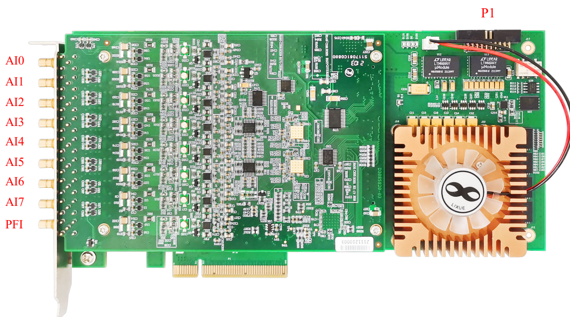
图 3-3-1 PCIe858xM 产品外观图
